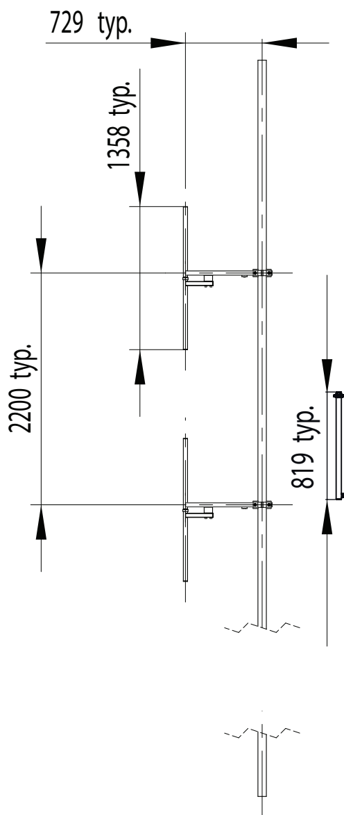
H-plane
