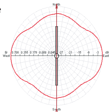
H-plane
